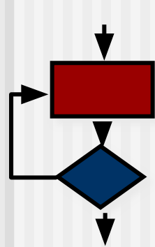
Simple loop
